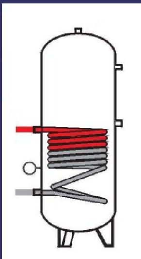
un serpentín
