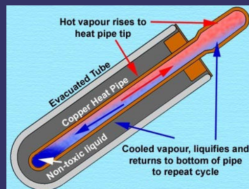
esquema do tubo de calor
