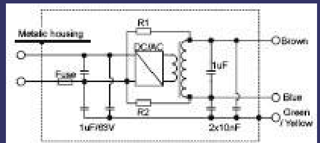
circuíto interno do inversor
