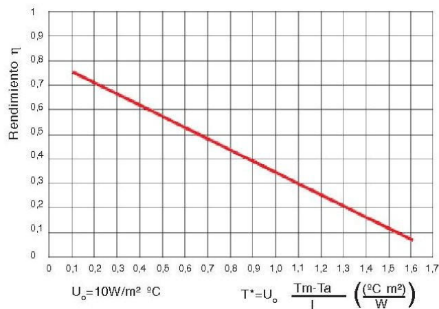
Curva de rendimiento
