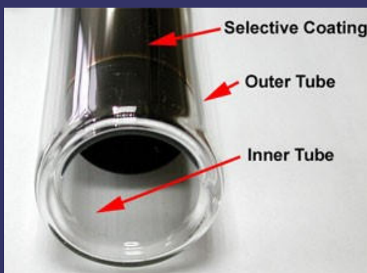
partes dun tubo de baleiro
